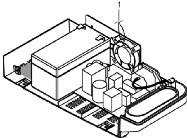
Figure 31: Fan Wires
